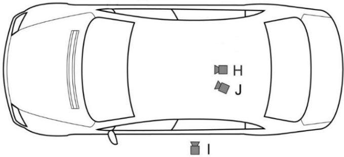
图 5 车载高速相机位置
