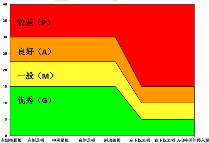
图 10 乘员舱侵入量等级评定
