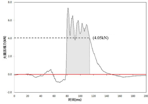
图 8 Hybrid III 50th 假人大腿冲量
