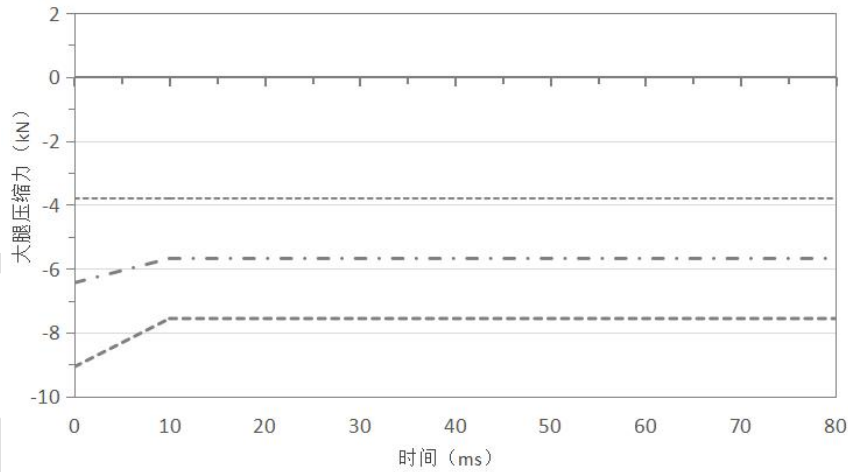
图 4 大腿压缩力累积曲线
