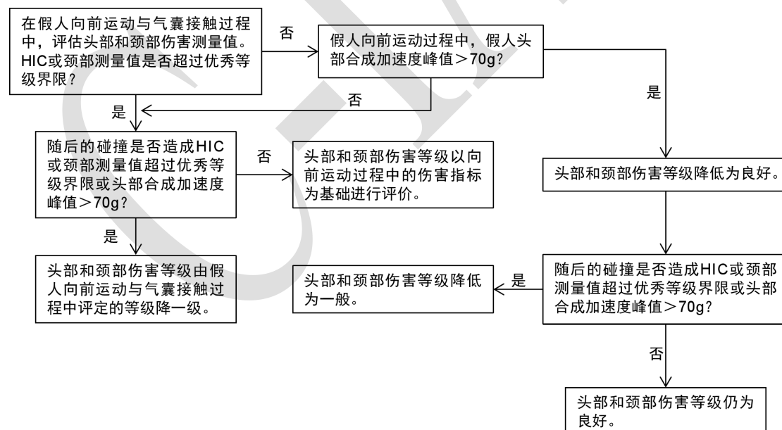
图 3 多次碰撞头部和颈部伤害评级流程图
