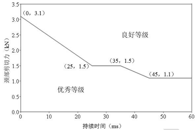
图 7 颈部剪切力 Fx 时间持续曲线
