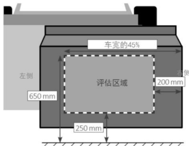
图 11 壁障蜂窝铝变形评估区域示意
