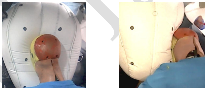
图 1 正面安全气囊不稳定接触（右图）示例
