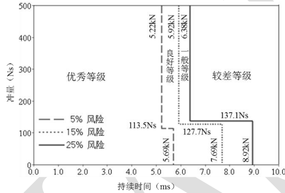
图 9 膝盖-大腿-髋部伤害风险 KTH
