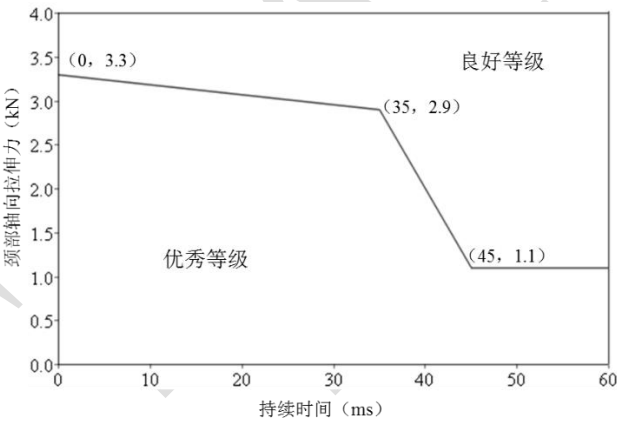
图 5 颈部拉伸力 F_z 时间持续曲线
