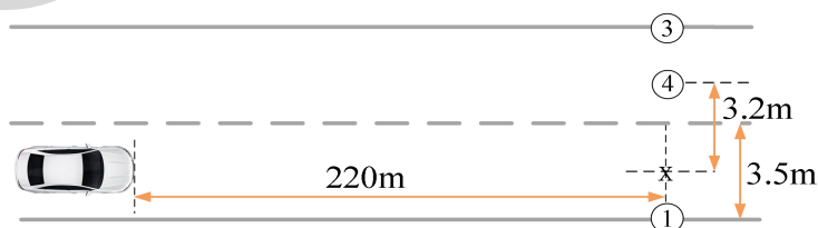
图 3 直道试验
