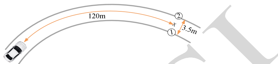
图 6 弯道试验
