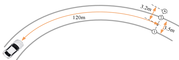
图 4 弯道试验
