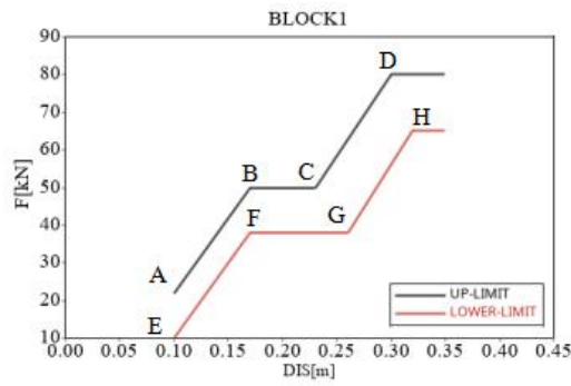
(a) 块 1 刚度特性要求
