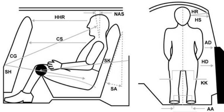
图 12 后排乘员假人空间位置测量示意图
