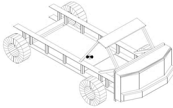
图4 移动变形壁障—AC-MDB
