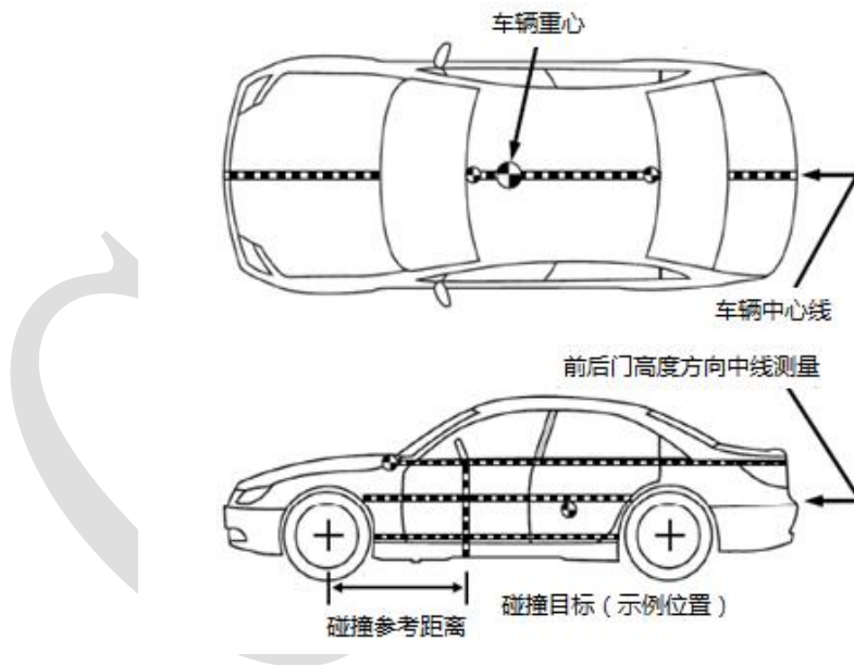
图 1 车辆外部表面标识
