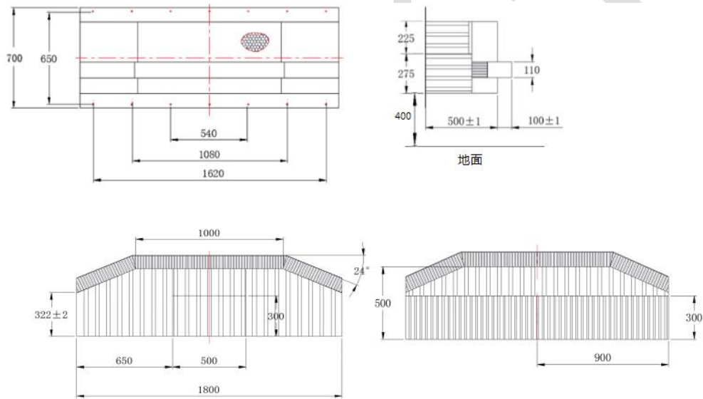
图5 碰撞块尺寸 (mm)
