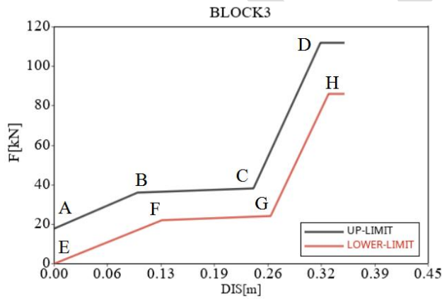
(c) 块 3 刚度特性要求
