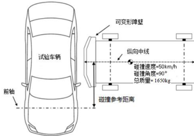
图 8 AC-MDB 与试验车辆
