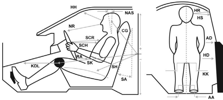
图 11 假人空间位置测量示意图
