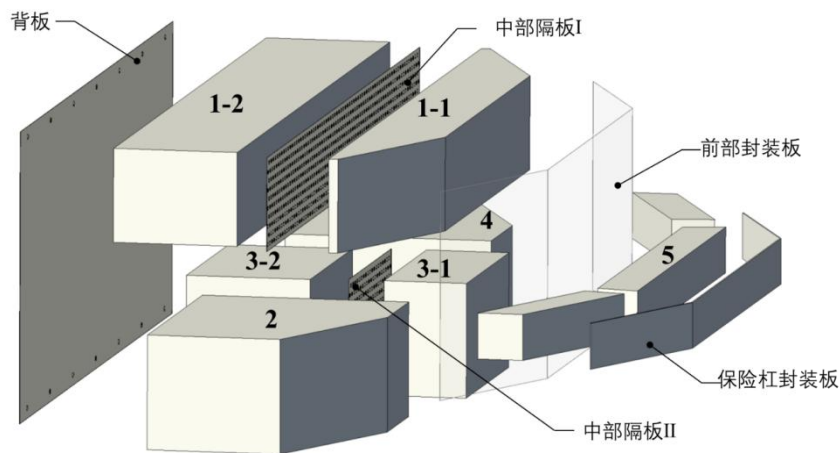
图6 碰撞块装配图
