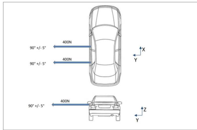
图 13 车门开启测量示意图
