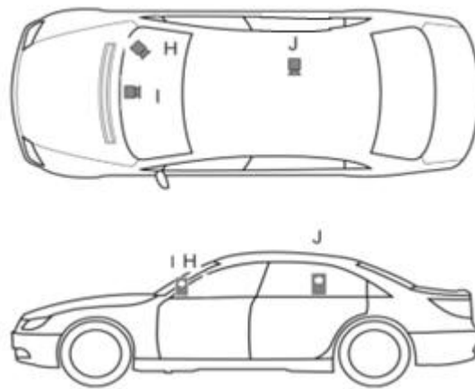
图 3 车载高速相机位置
