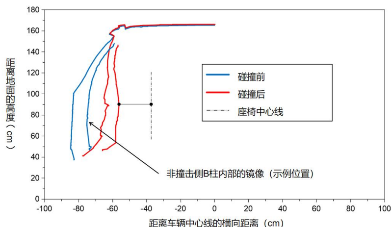
图 9 B 柱垂直剖面示例
