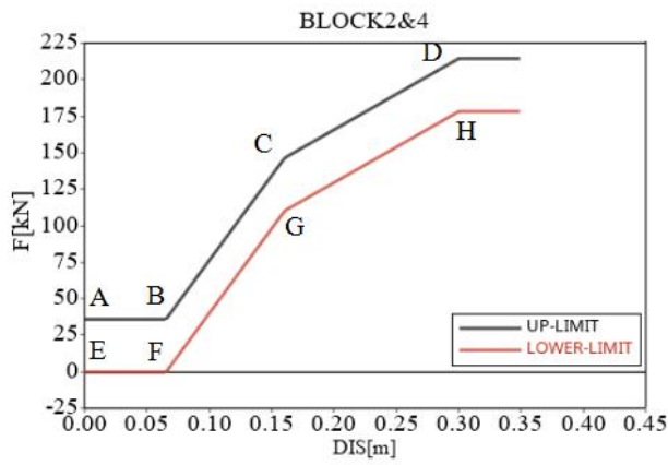
(b) 块 2 和块 4 刚度特性要求
